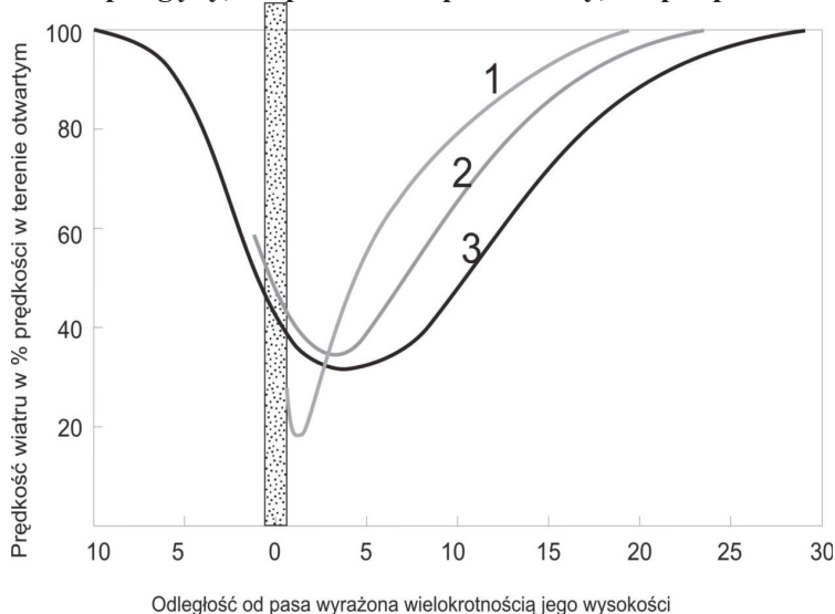
Rysunek 2. Prędkość wiatru w zależności od odległości od pasa zadrzewień wyrażona w procentach prędkości na otwartym terenie: 1 – pas gęsty, 2 – pas średnio przewiewny, 3 – pas przewiewny
